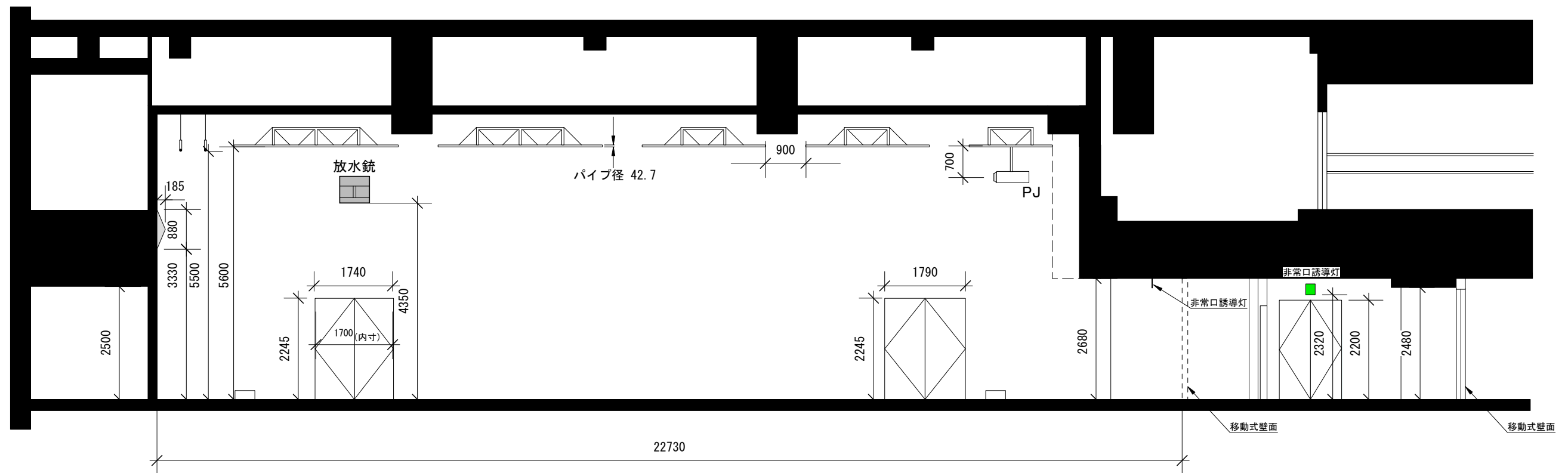
■ B 立面図
